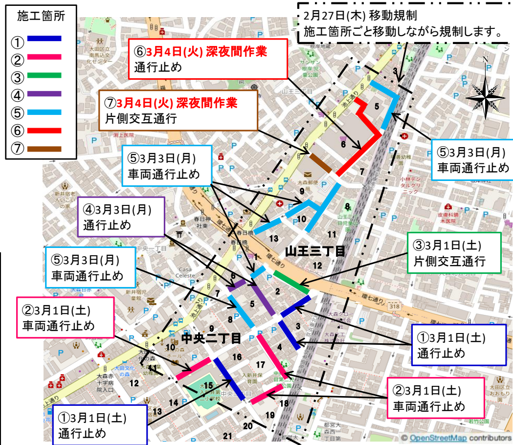
本復旧工 アスファルト舗装を新しく舗装する
