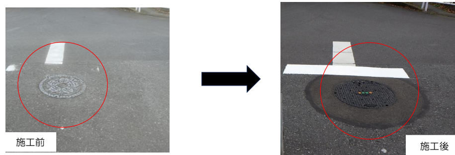
人孔上部補修工：劣化したマンホールを新しい蓋・鉄枠へ取替
