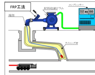
内面被覆工：道路を掘削しないで、古い管の耐久性を向上させる工法
