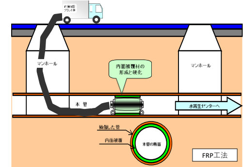
内面被覆工事にて補修した本管
