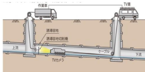
上流・下流のマンホールへ削孔機・TVカメラにて端部切断を行います。
