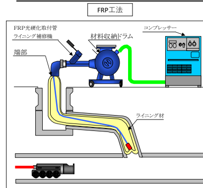
内面被覆工事にて補修した取付管
