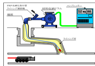
内面被覆工事にて補修した取付管
