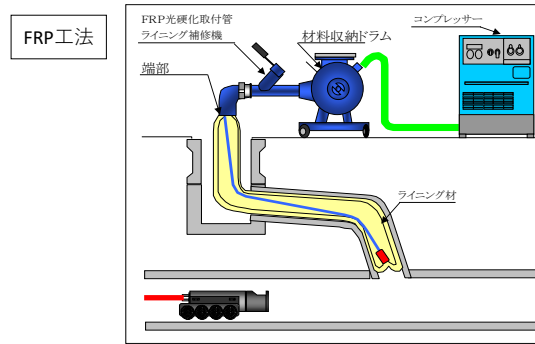
内面被覆工事にて補修した取付管
