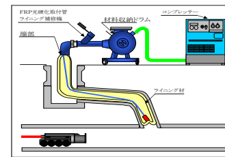
内面被覆工事にて補修した取付管
