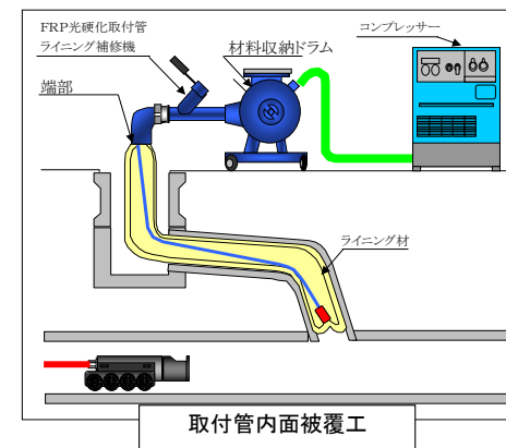
12/14 内面被覆工
