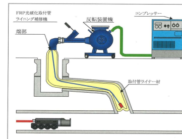
内面被覆工にて補修した取付管
