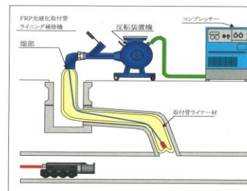
内面被覆工にて補修した取付管
