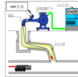
内面被覆工事にて補修した取付管
