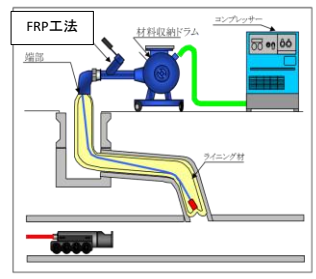
内面被覆工事にて補修した取付管
