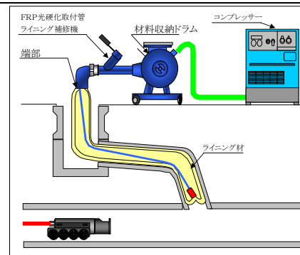
内面被覆工事にて補修した取付管
