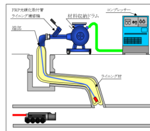
損傷した既設の下水道管きょ内部を非開削で施工
