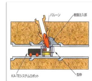
不要となった取付管内に泡モルタル等を充填する非開削で施工
