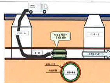
内面被覆工事にて 補修した本管
