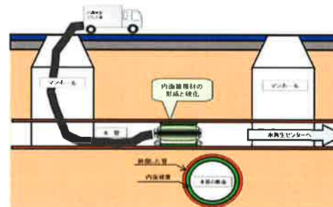
内面被覆工事にて補修した本管
